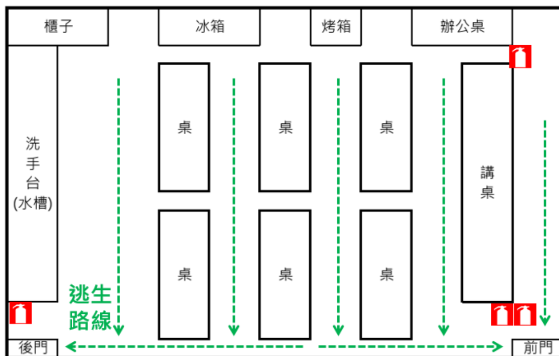
平面圖
