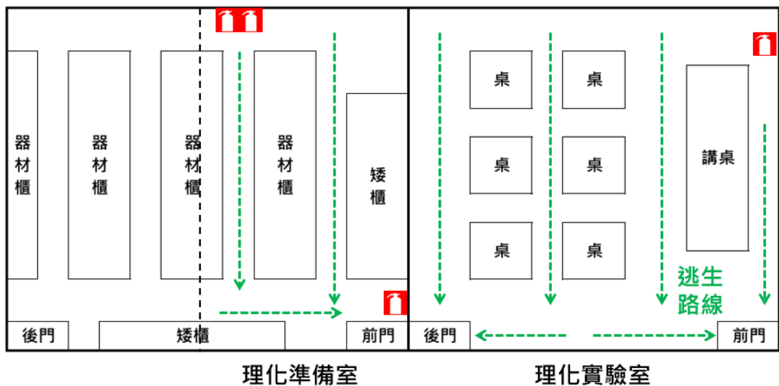
平面圖
